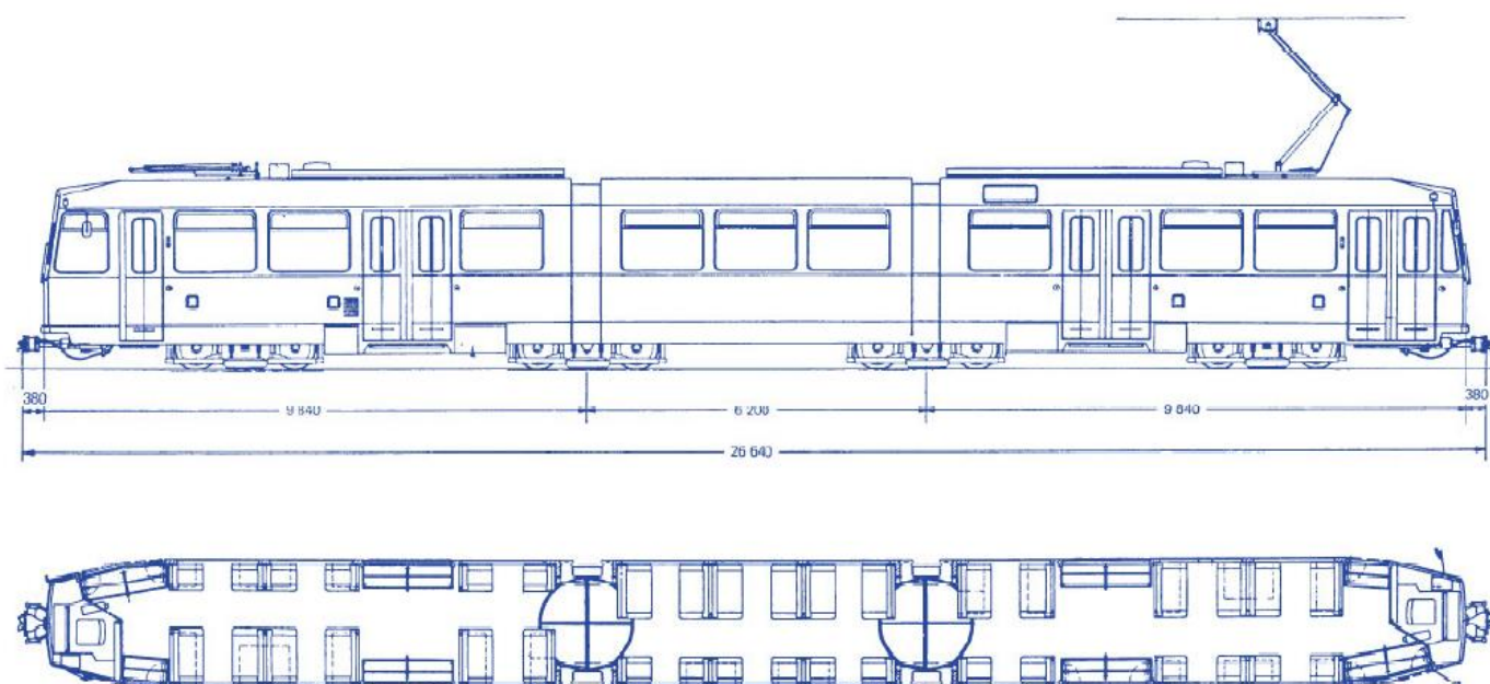
Fig.12. Tramvai M8S
