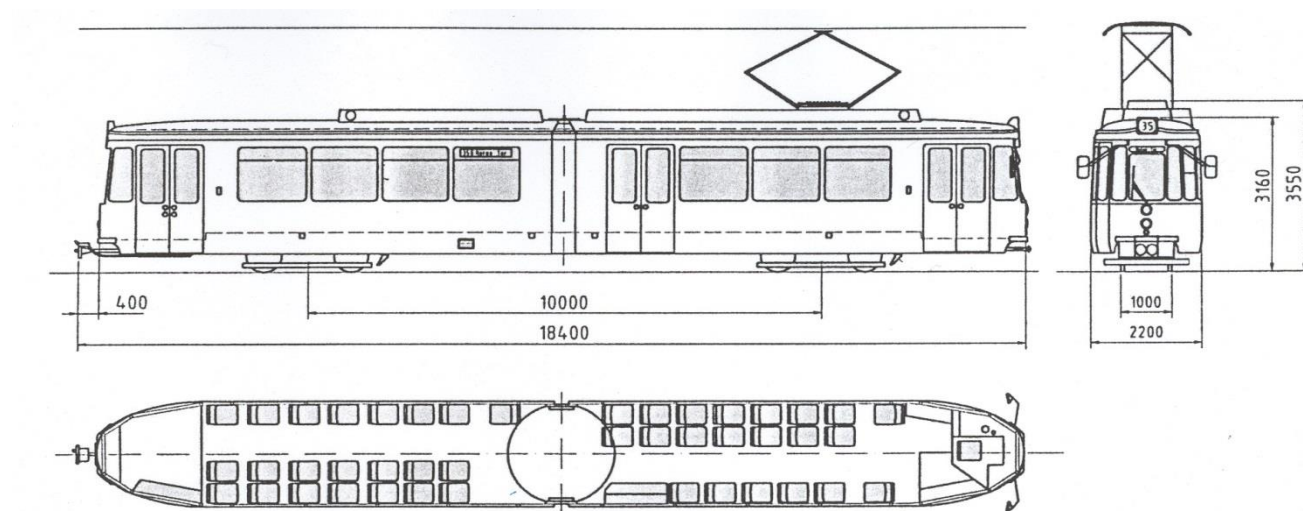
Fig.8. Tramvai GT4
