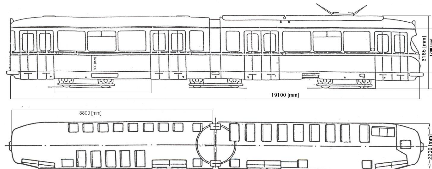
Fig.9. Tramvai GT6
